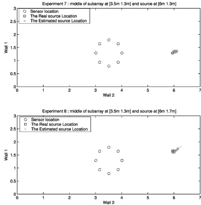
Fig. 24. Circular subarray: Experiments 7 and 8.
